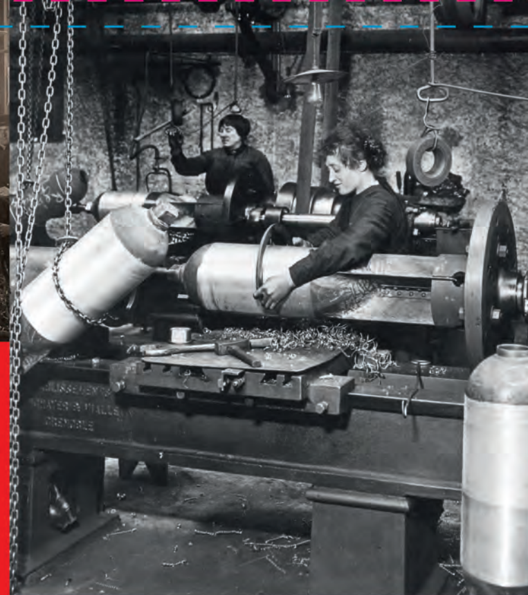
Tournage des bombes effectué par deux ouvrières des Établissements Bouchayer-et-Viallet, Grenoble, 1914-1918. Collection Archives départementales de l'Isère
